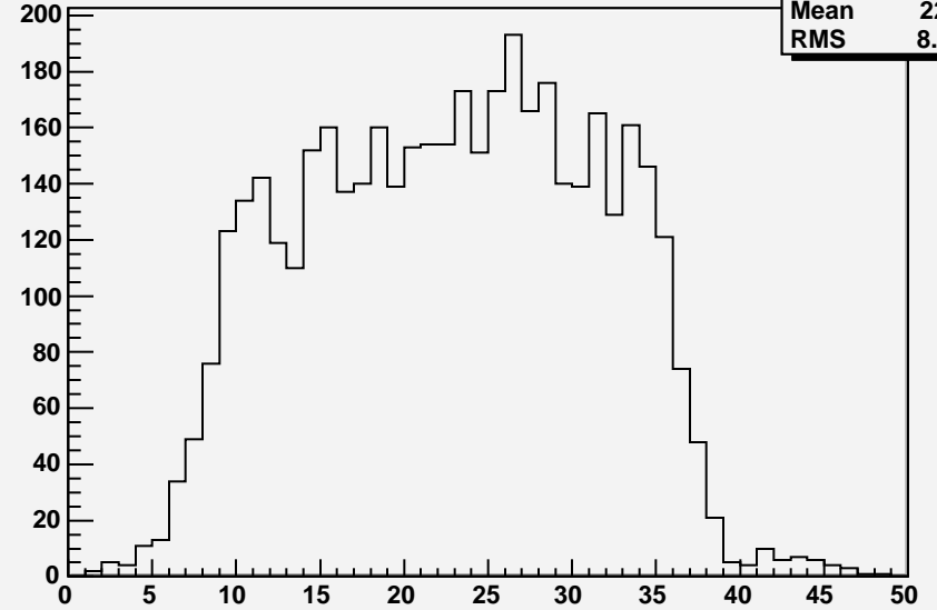
Number per detector of V1 Right
