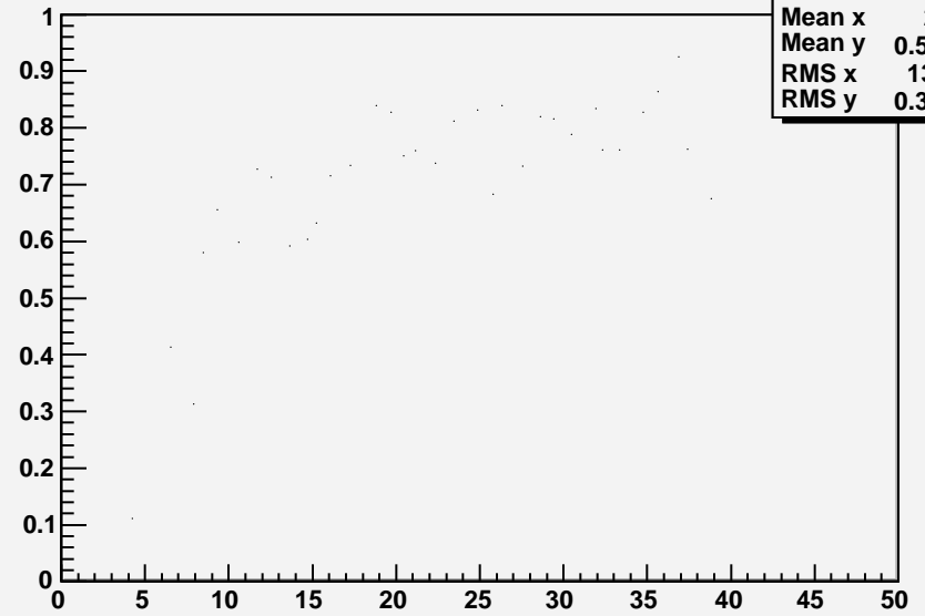
Efficiencies per detector of V1 Right
