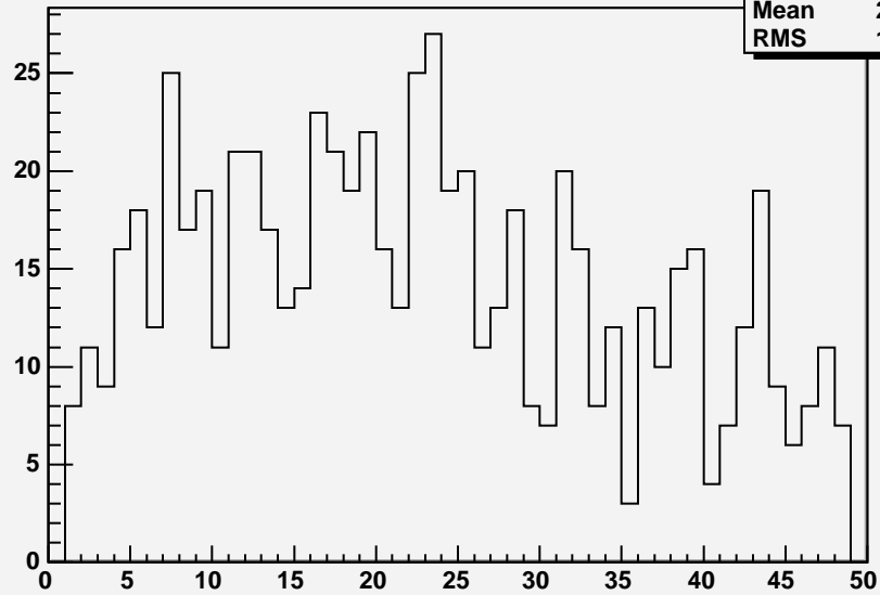
Number per detector of V1 Left
