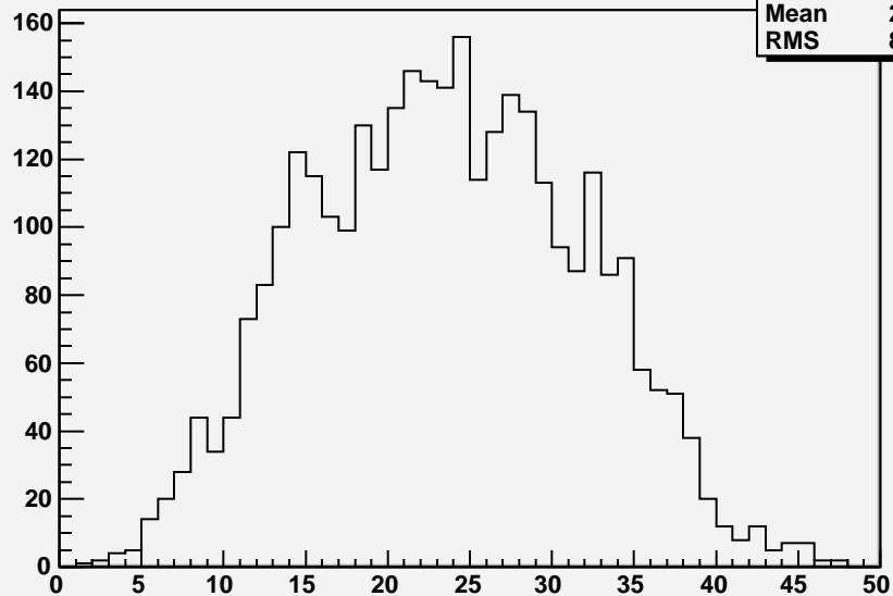
Number per detector of V2 Left
