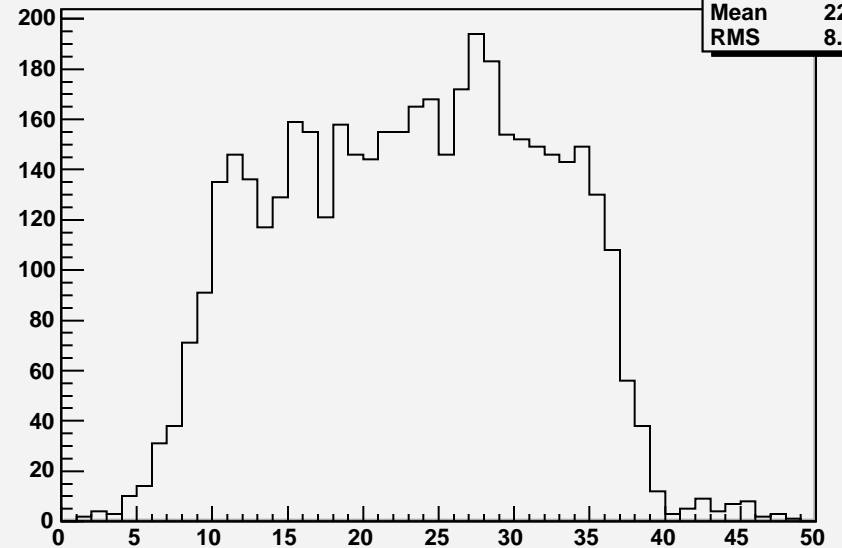
Number per detector of V2 Right
