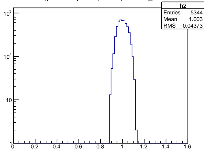
(pr11.e + pr12.e) / L.tr.p of cut_e
