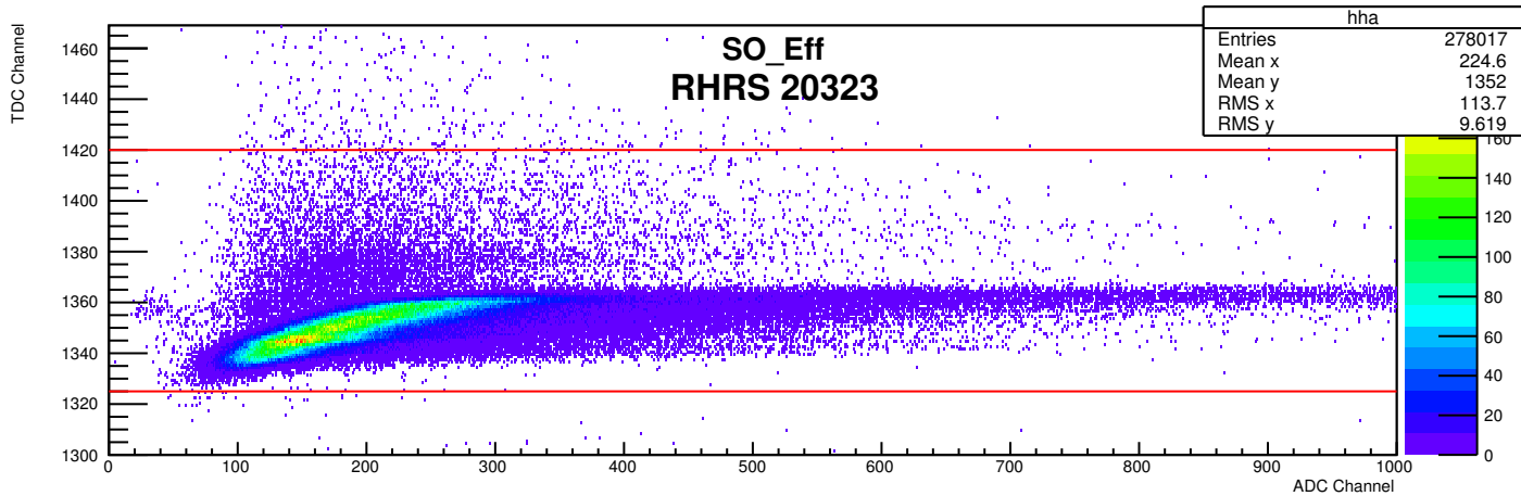
s0-A TDC vs. ADC:All Hits
