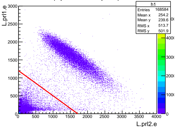
cut3: -0.06 < L.tr.vz < 0.06
