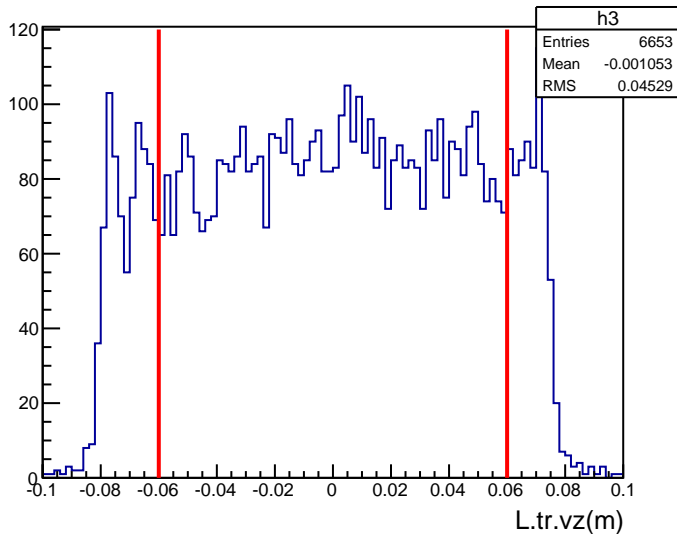
cut3: -0.06 < L.tr.vz < 0.06
