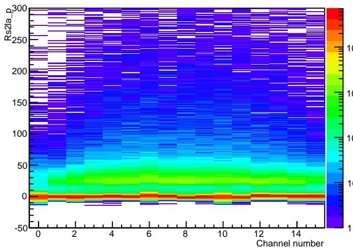
Rs2la_p0-15
