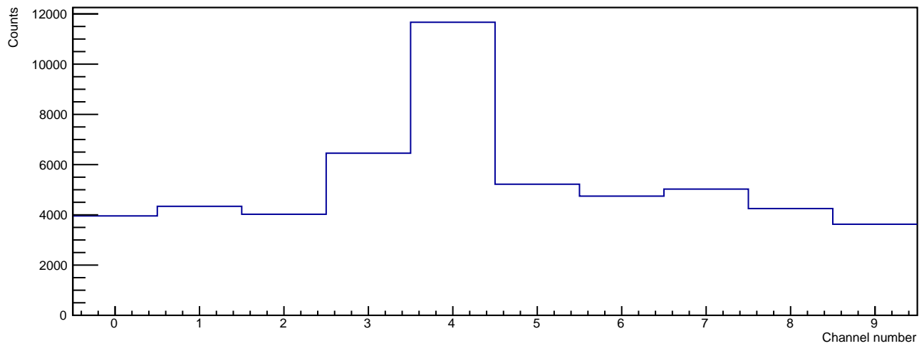
Rcert0-9_counts
