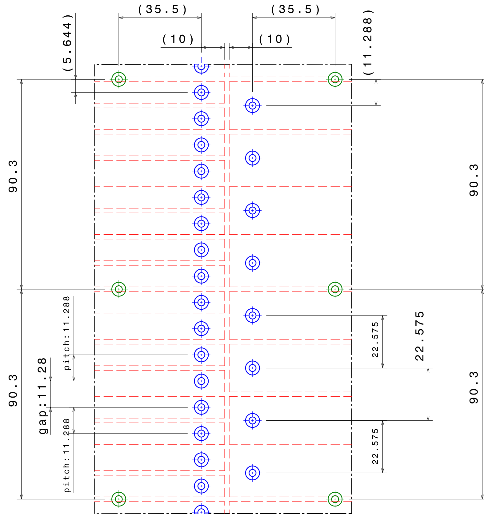
Detail A Scale: 1:1
