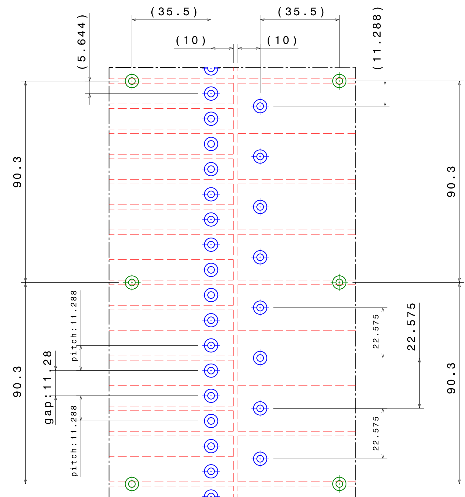
Detail A Scale: 2:1
