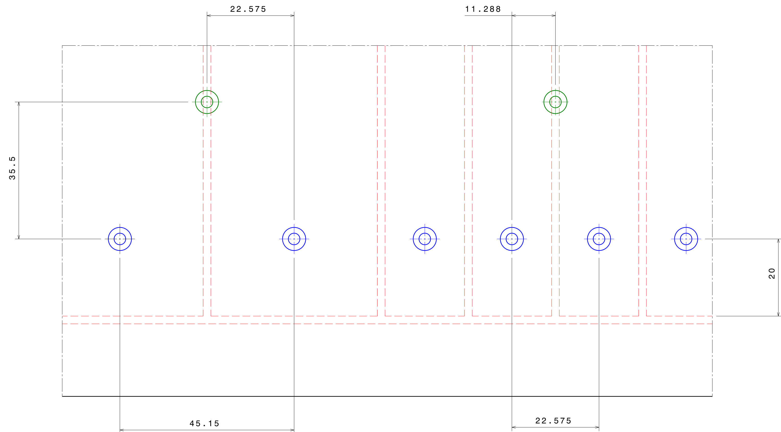
Detail A Scale : 2:1
