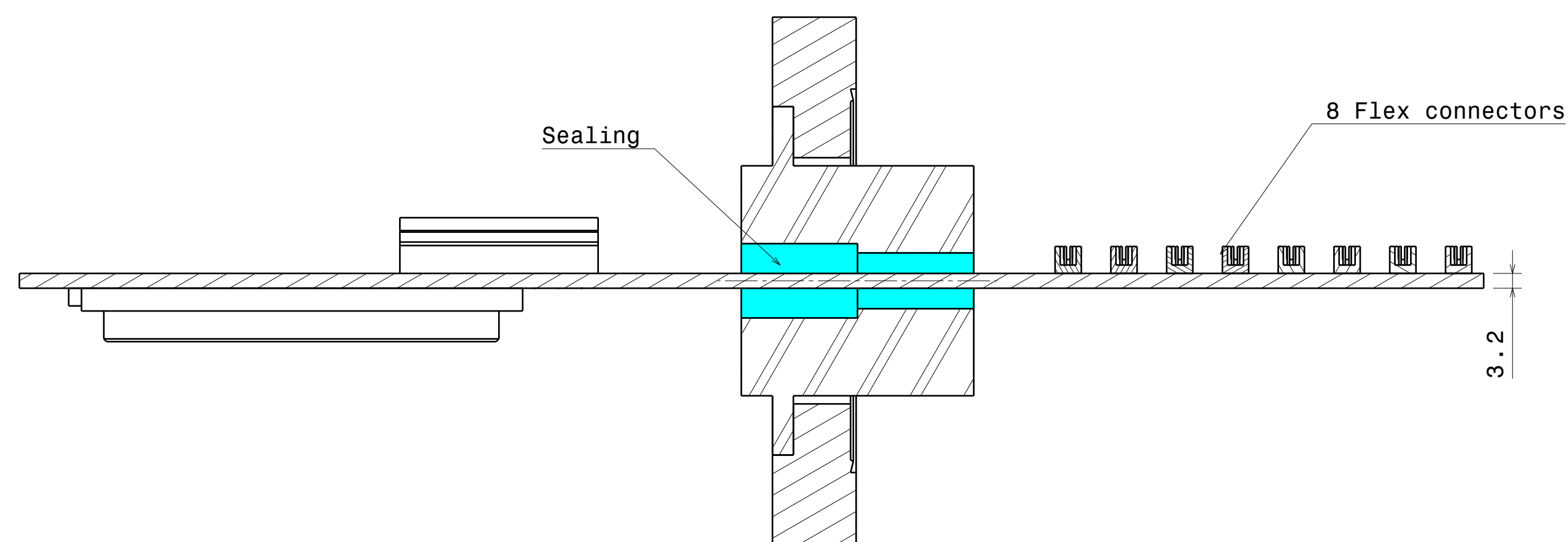
Coupe A-A
