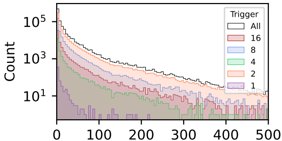
Shower_t
