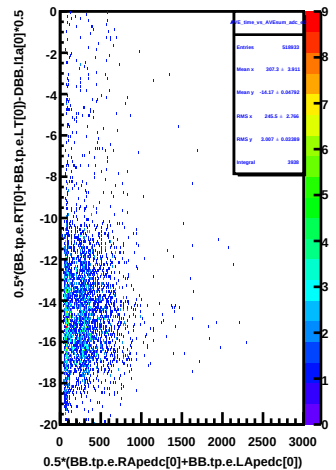
AVE_time_vs_AVEsum_adc_e0
