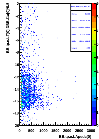
Left_time_vs_adc_e0
