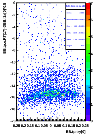
Right_time_vs_try_e17
