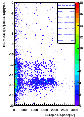
Right_time_vs_adc_e17
