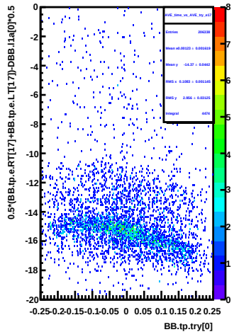
AVE_time_vs_AVE_try_e17
