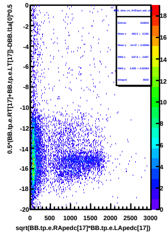
AVE_time_vs_AVEsqr_adc_e17
