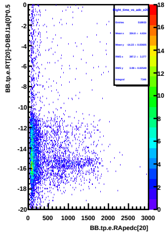
Right_time_vs_adc_e20
