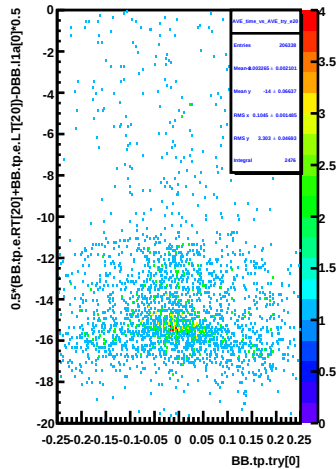
AVE_time_vs_AVE_try_e20
