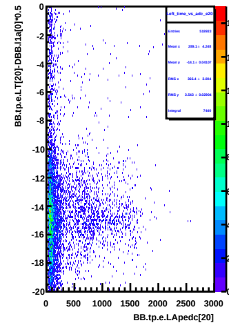
Left_time_vs_adc_e20
