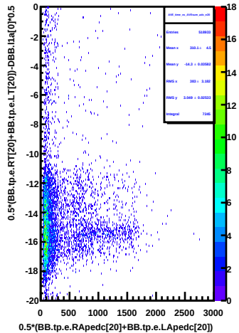
AVE_time_vs_AVEsum_adc_e20
