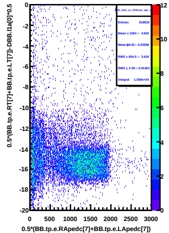
AVE_time_vs_AVEsum_adc_e7
