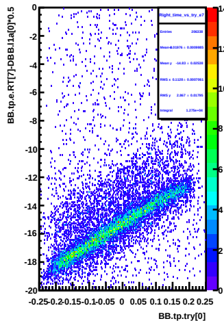
Right_time_vs_try_e7
