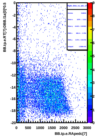
Right_time_vs_adc_e7
