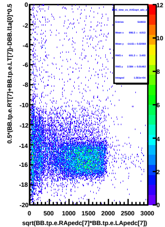
AVE_time_vs_AVEsqrt_adc_e7
