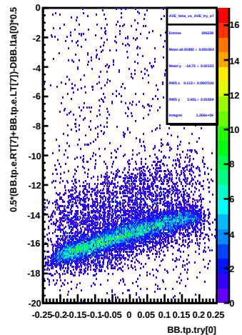
AVE_time_vs_AVE_try_e7
