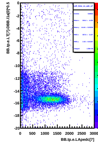
Left_time_vs_adc_e7
