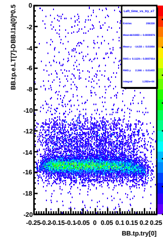
Left_time_vs_try_e7
