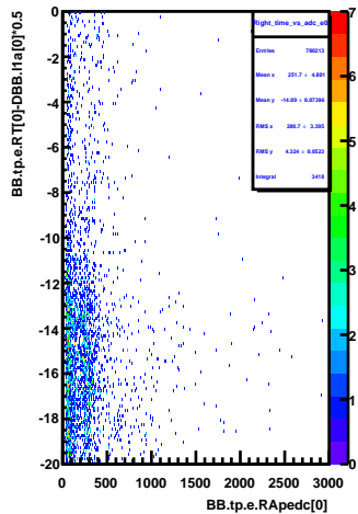
Right_time_vs_adc_e0
