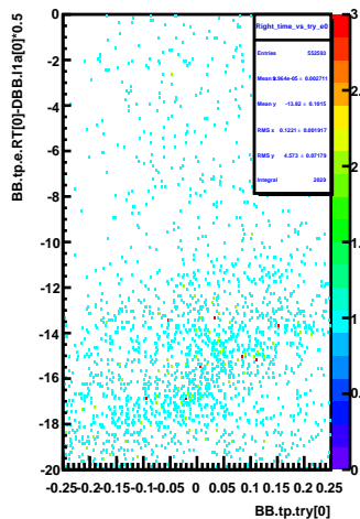
Right_time_vs_try_e0
