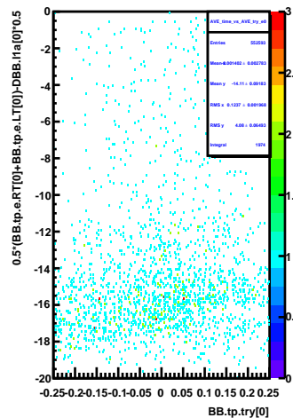
AVE_time_vs_AVE_try_e0
