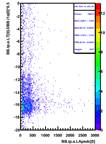
Left_time_vs_adc_e0
