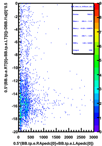
AVE_time_vs_AVEsum_adc_e0
