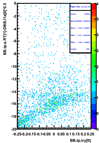
Right_time_vs_try_e1
