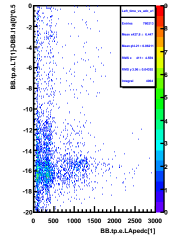
Left_time_vs_adc_e1
