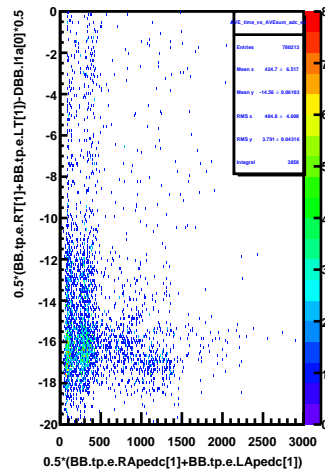
AVE_time_vs_AVEsum_adc_e1
