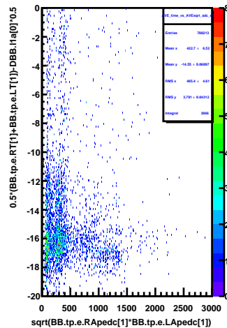
AVE_time_vs_AVEsqrt_adc_e1
