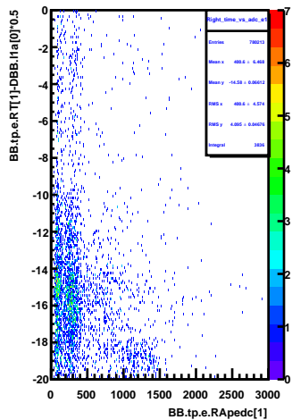
Right_time_vs_adc_e1
