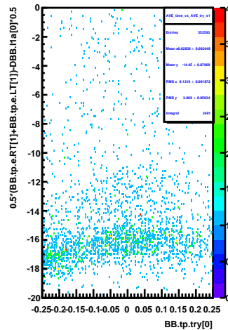
AVE_time_vs_AVE_try_e1
