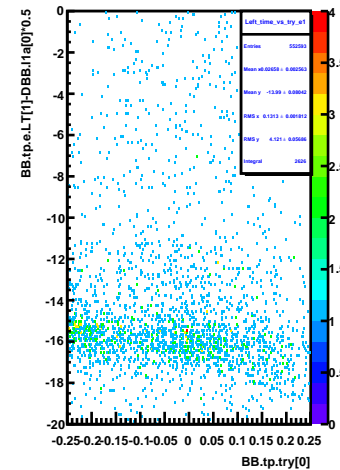
Left_time_vs_try_e1
