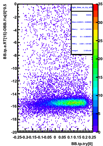
Right_time_vs_try_e15
