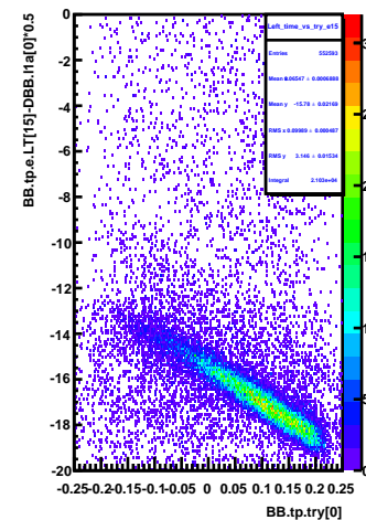
Left_time_vs_try_e15
