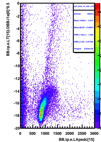
Left_time_vs_adc_e15
