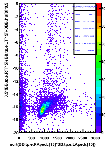
AVE_time_vs_AVEsqrt_adc_e15
