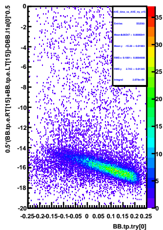
AVE_time_vs_AVE_try_e15
