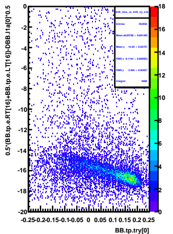
AVE_time_vs_AVE_try_e16
