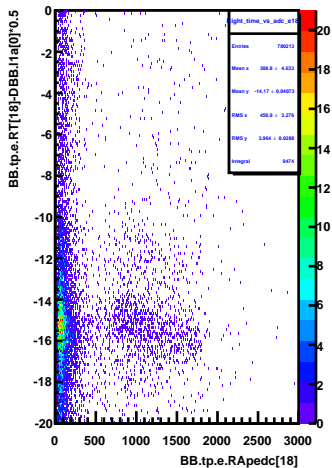
Right_time_vs_adc_e18
