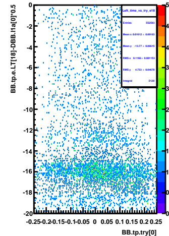
Left_time_vs_try_e18
