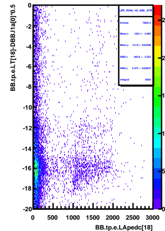
Left_time_vs_adc_e18
