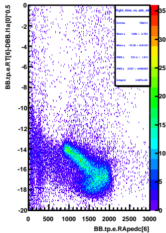
Right_time_vs_adc_e6
