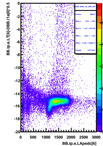
Left_time_vs_adc_e6
