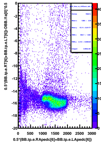
AVE_time_vs_AVEsum_adc_e6
