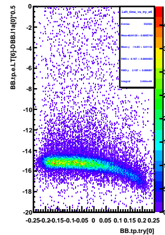
Left_time_vs_try_e6
