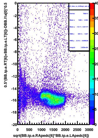
AVE_time_vs_AVEsqrt_adc_e6
