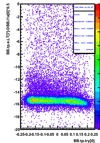
Left_time_vs_try_e7
