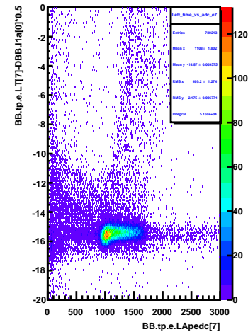
Left_time_vs_adc_e7
