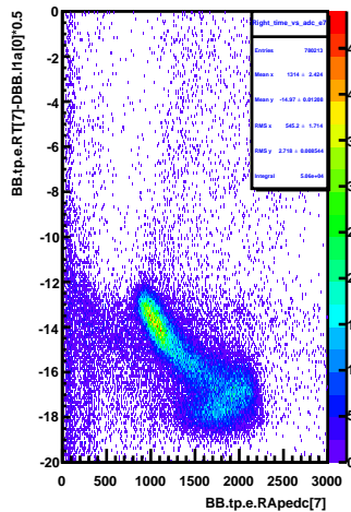
Right_time_vs_adc_e7
