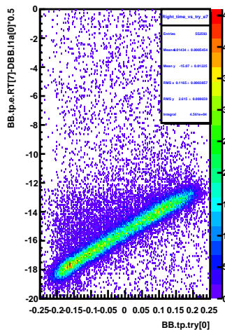
Right_time_vs_try_e7
