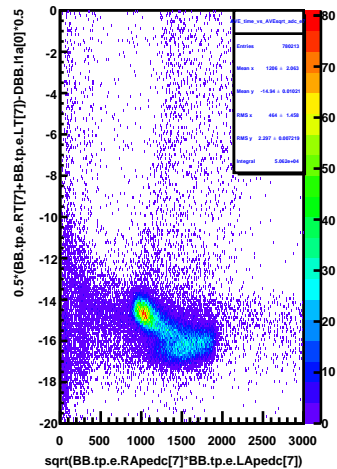
AVE_time_vs_AVEsqrt_adc_e7
