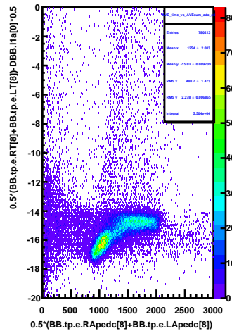
AVE_time_vs_AVEsum_adc_e8
