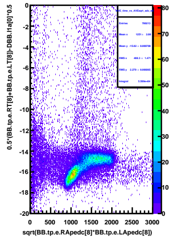
AVE_time_vs_AVEsqrt_adc_e8
