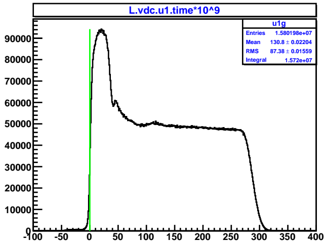
L.vdc.u1.time*10^9
