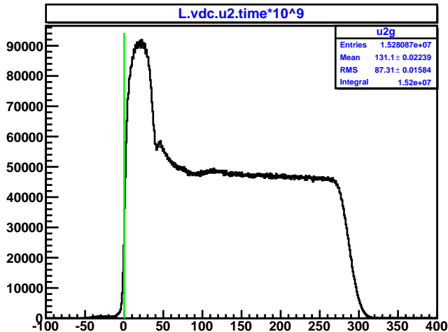
L.vdc.u2.time*10^9
