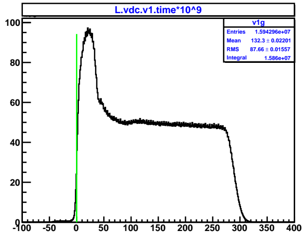
L.vdc.v1.time*10^9
