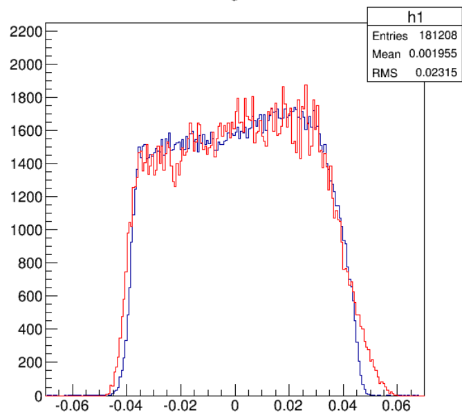
\delta
