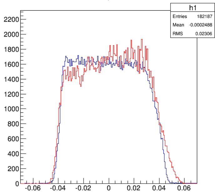
\delta
