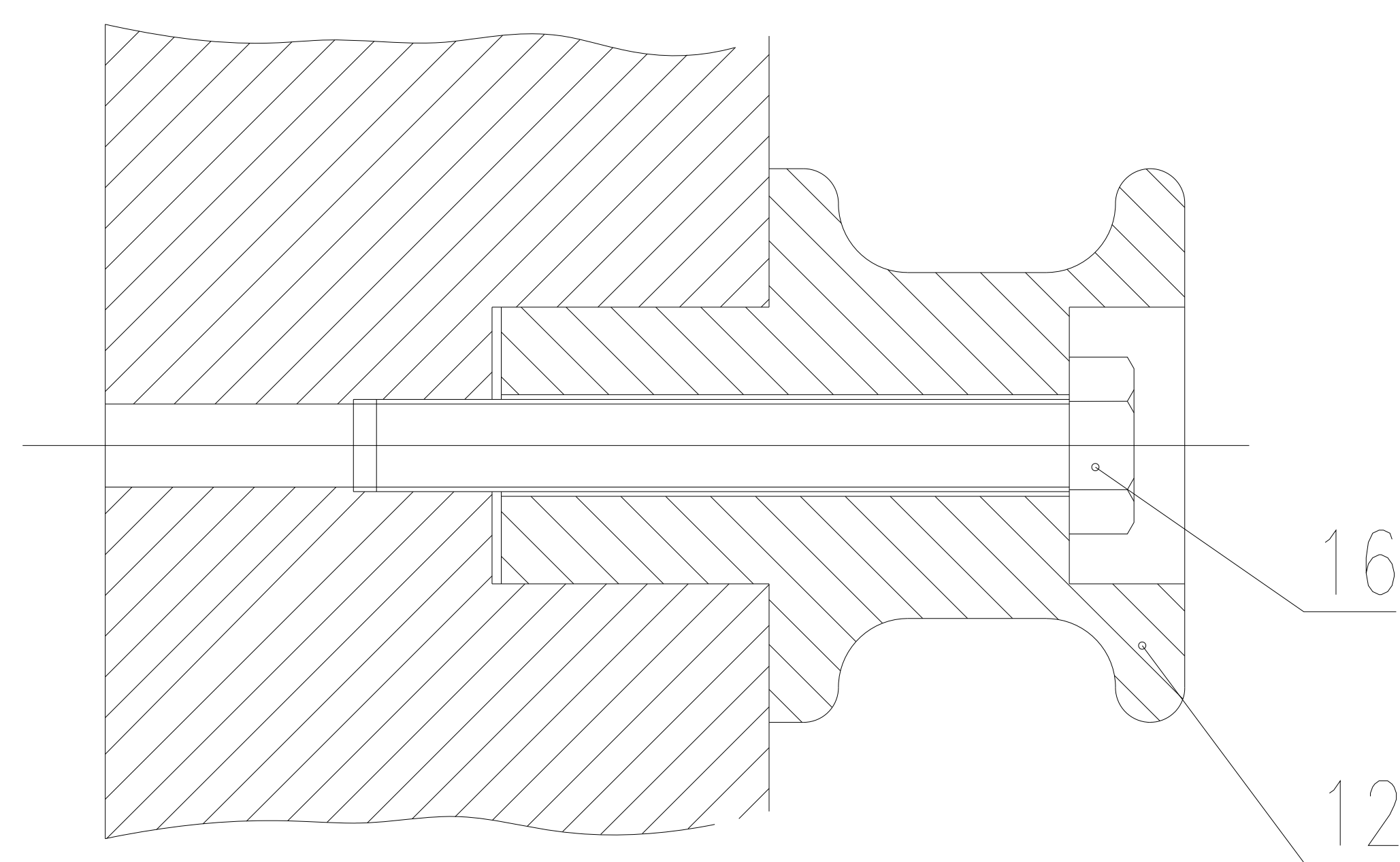
T-T 1:2 sheet 1
