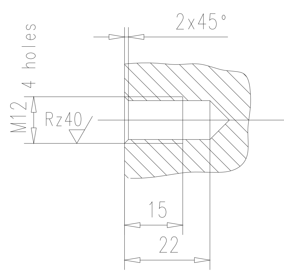
O-O 1:1
