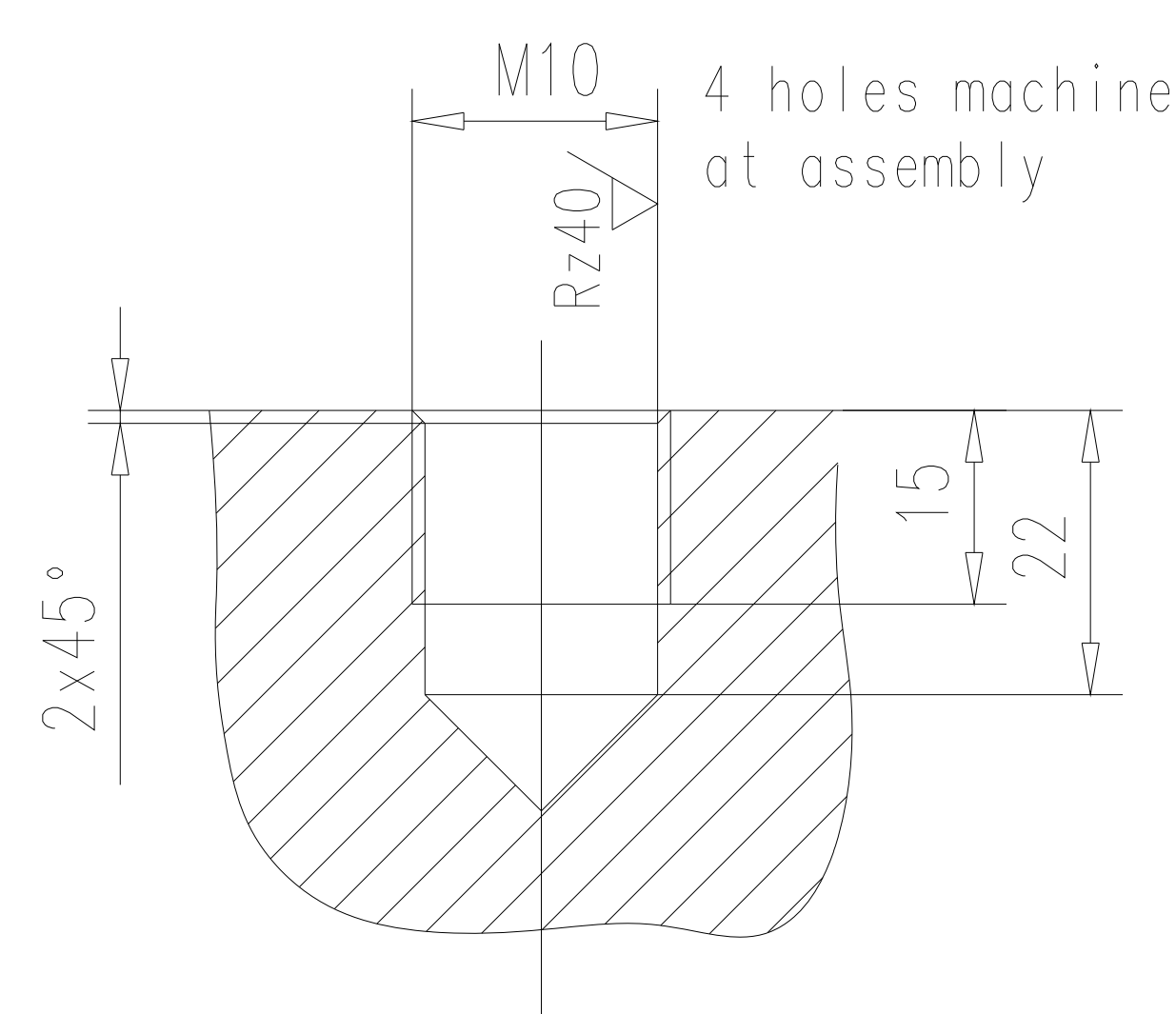
M-M 1:1 sheet 1
