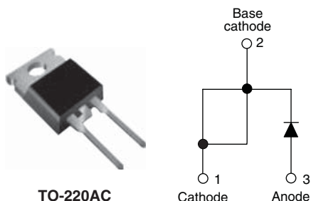
TO-220AC
