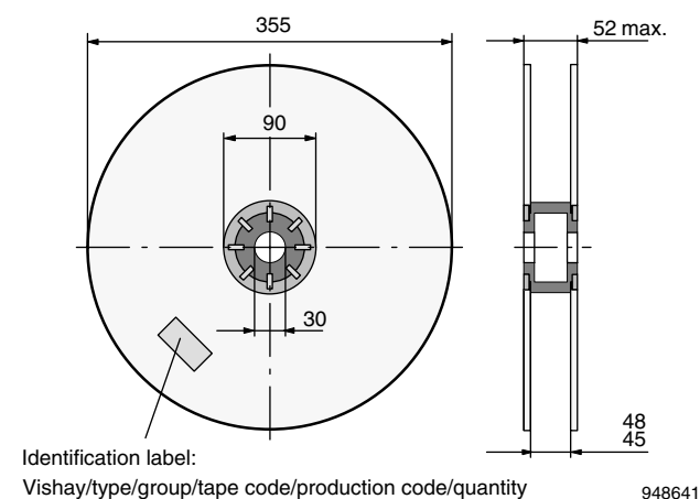
Fig. 16 - Reel Dimensions
