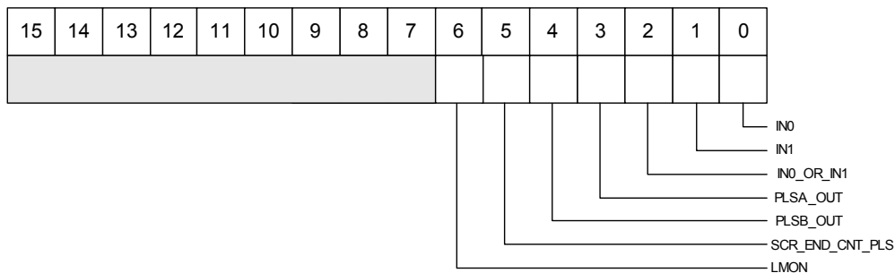
Fig. 2.9: Input register
