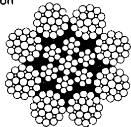
8x25 Filler, IWRC
