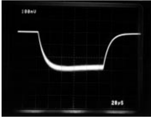
(a) R_L=20k\Omega
