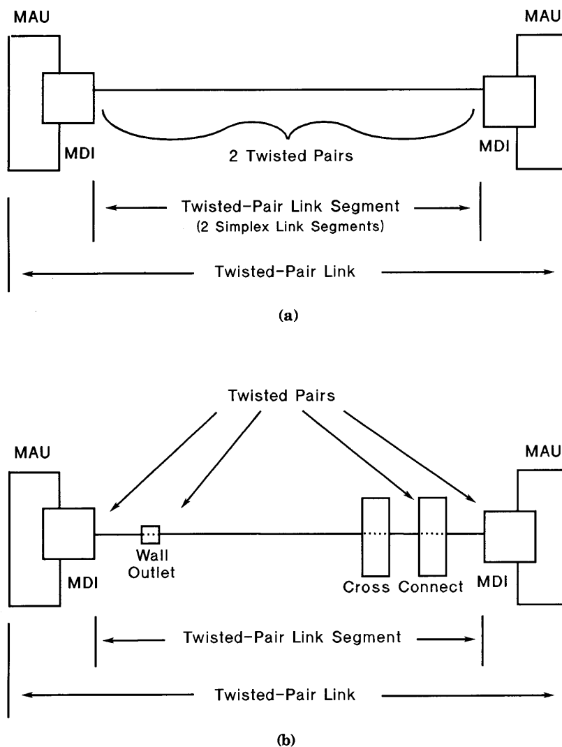
Figure 14-2—Twisted-pair link
