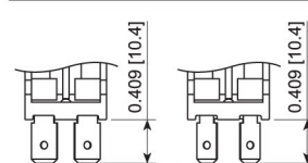
6.3mm Tab
