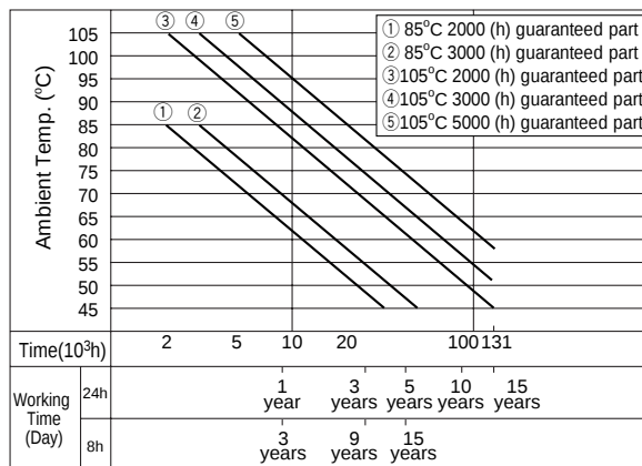
Fig. 2-15 Life Estimation Table
