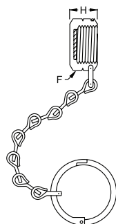
CGA Cap 320-350 & 660-705
