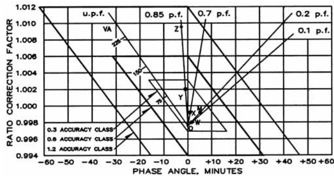
Circle Diagram
