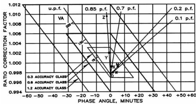
Circle Diagram
