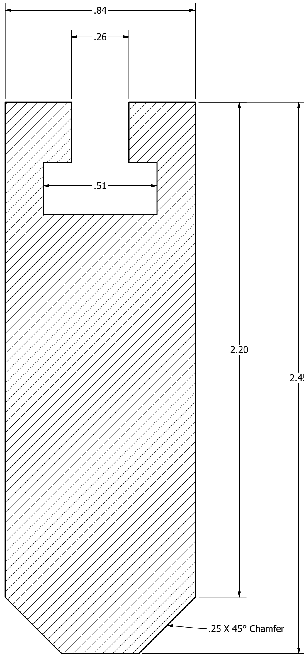
SECTION A-A SCALE 4 : 1
