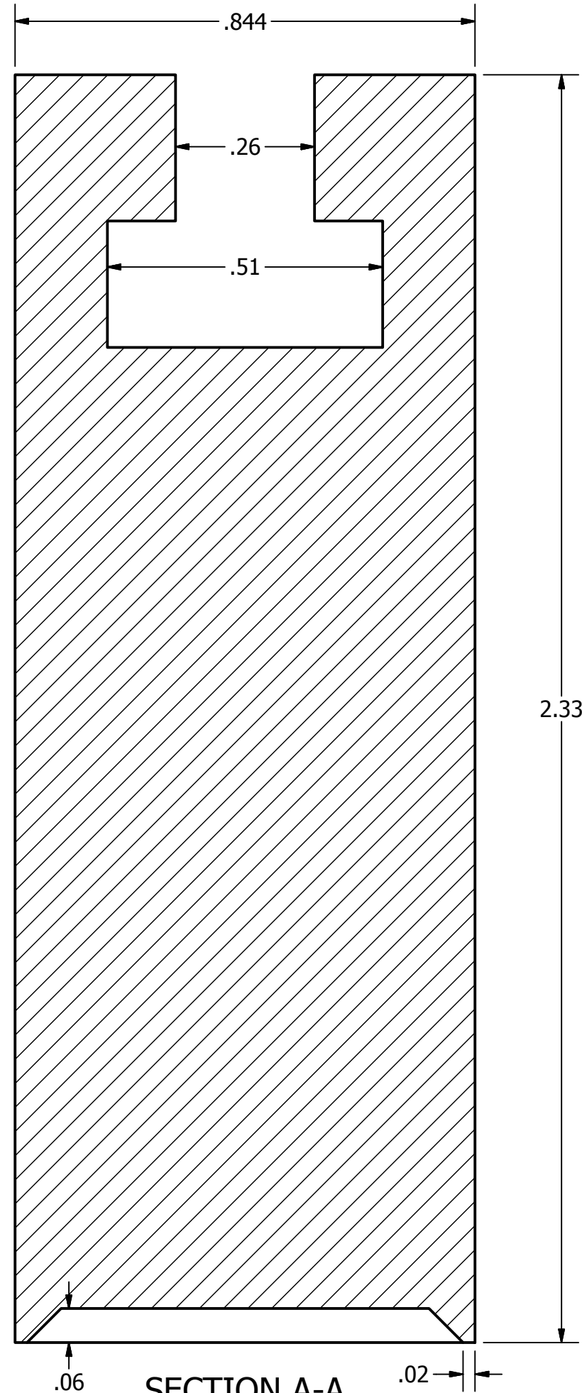
SECTION A-A SCALE 4 : 1
