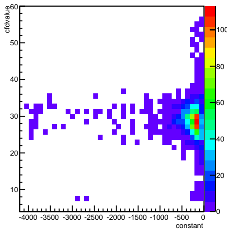
HV=3.56kV {constant<-50}
