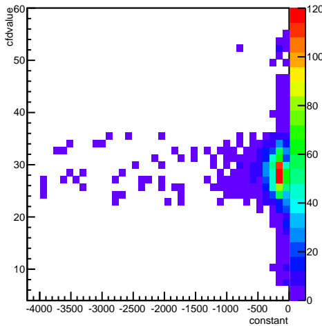
HV=3.47kV {constant<-50}
