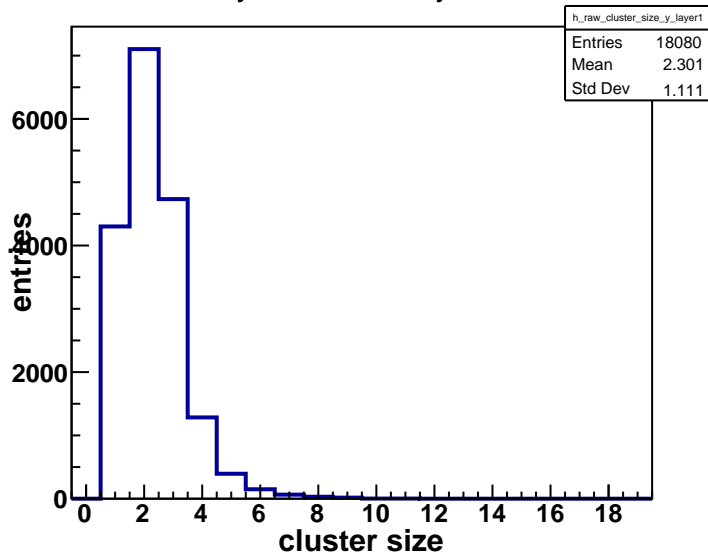
y cluster size layer1
