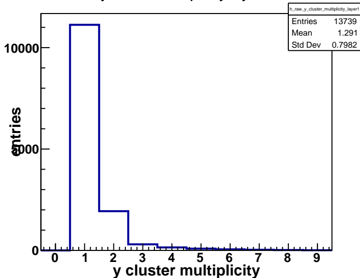
y cluster multiplicity layer 1
