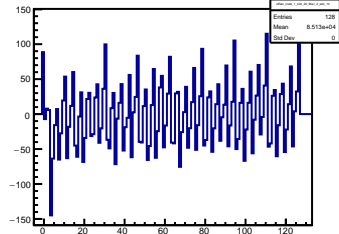
offset_crate_1_slot_20_fiber_2_adc_12
