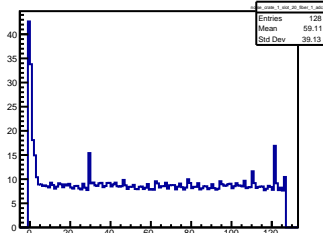
noise_crate_1_slot_20_fiber_1_adc_6
