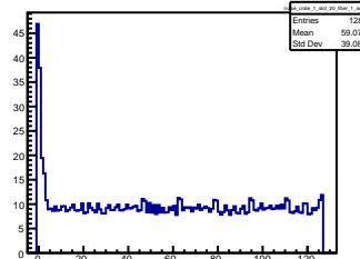
noise_crate_1_slot_20_fiber_1_adc_3
