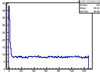
noise_crate_1_slot_20_fiber_7_adc_11
