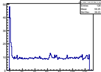
noise_crate_1_slot_20_fiber_4_adc_1
