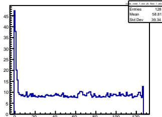
noise_crate_1_slot_20_fiber_1_adc_11
