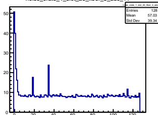
noise_crate_1_slot_20_fiber_3_adc_11
