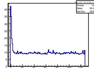
noise_crate_1_slot_20_fiber_4_adc_7
