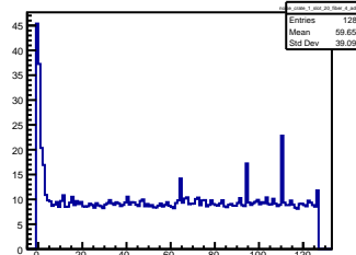
noise_crate_1_slot_20_fiber_4_adc_2
