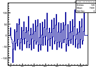
offset_crate_1_slot_20_fiber_6_adc_8
