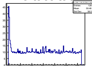
noise_crate_1_slot_20_fiber_4_adc_9
