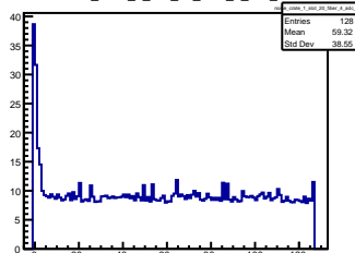
noise_crate_1_slot_20_fiber_4_adc_13
