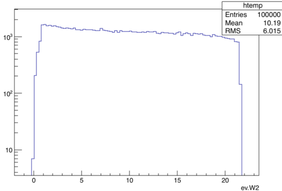
ev.W2
