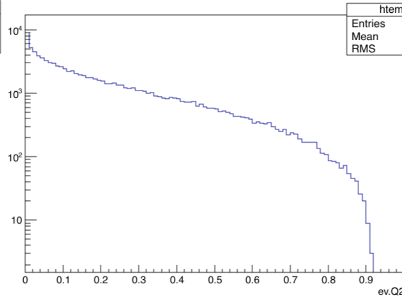
ev.Q2
